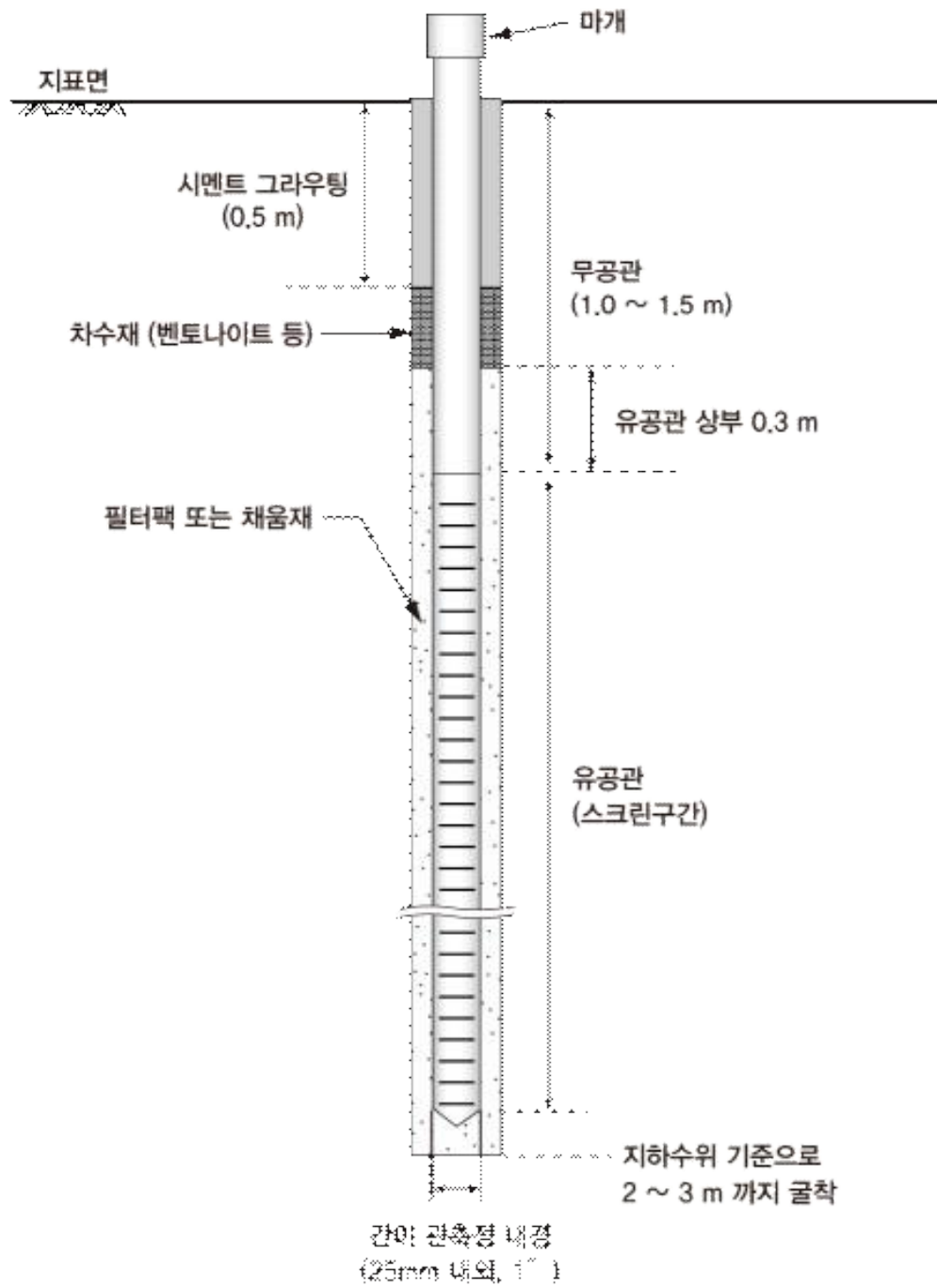
[별표 4] 간이 관측정 구조 기본도
